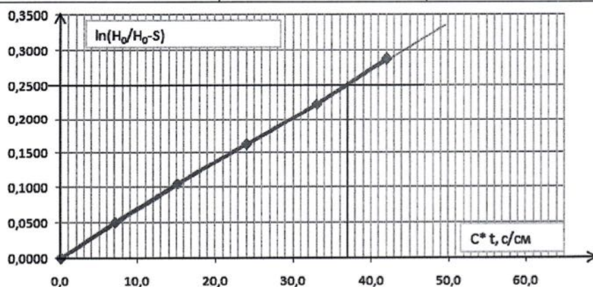
Рис. 1 График для определения коэффициента фильтрации песчаных грунтов, применяемых в дорожном и аэродромном строительстве.
